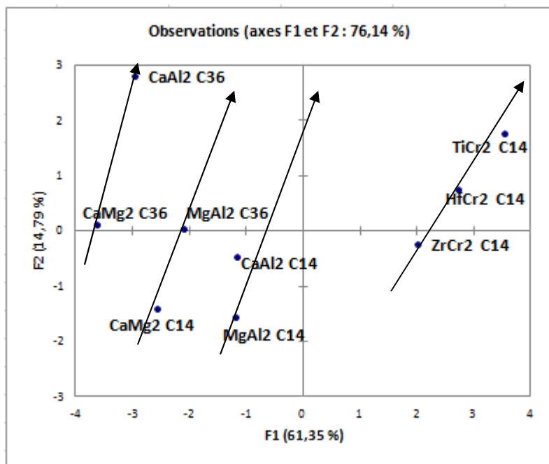
Figure (III-5) : graphe des observations des matériaux cristallisant dans la C14 et la C36.
