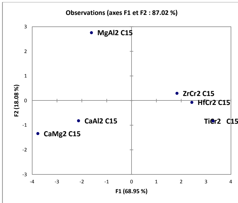
Figure (III-4) : graphe des observations des matériaux cristallisant dans la C15.
