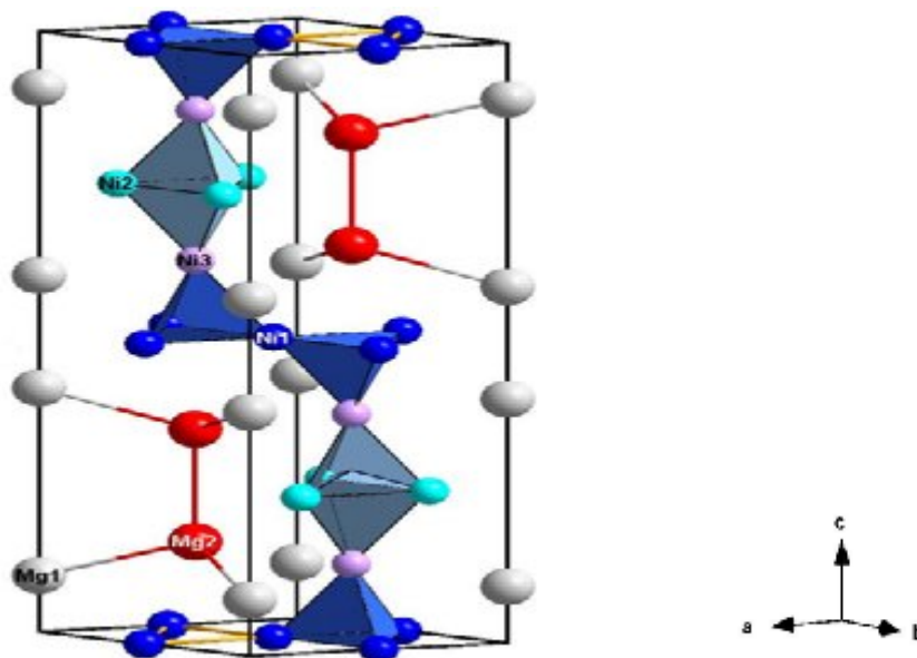
Fig.3 Structure type MgNi_2 ou C36
