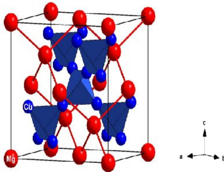
Fig.1 : Structure type MgCu_2 ou C15.
