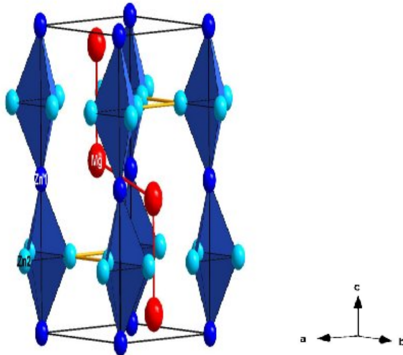
Fig.2 Structure type MgZn_2 ou C14.
