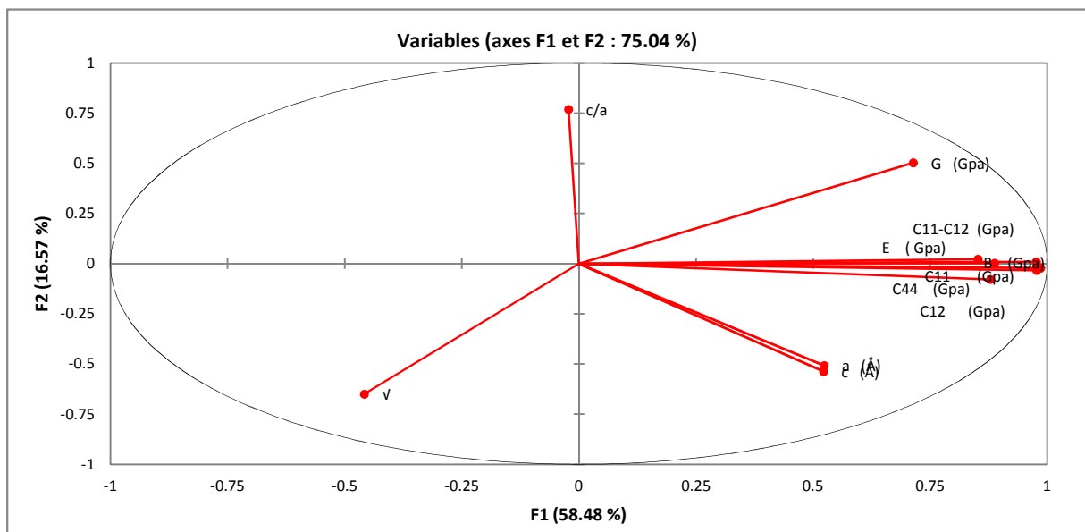
Figure (III-1) : graphe des propriétés (loading plot).
