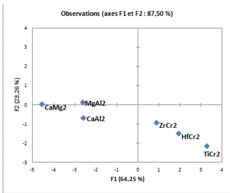
Figure (III-3) : graphe des observations des matériaux cristallisant dans la C14.
